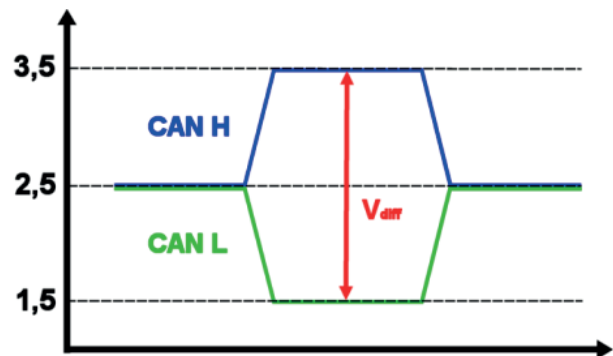
Figura 26: Segnale CAN alta e bassa velocità
