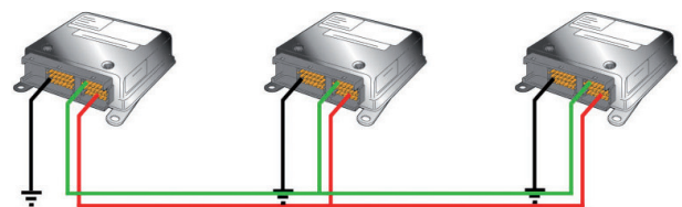
Figura 15: Collegamento bifilare
