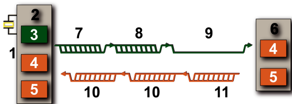
Figura 21: Esempio di scambio dati tra nodo slave e master
