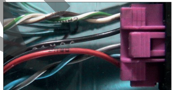
Figura 25: Doppino twistato di collegamento CAN
