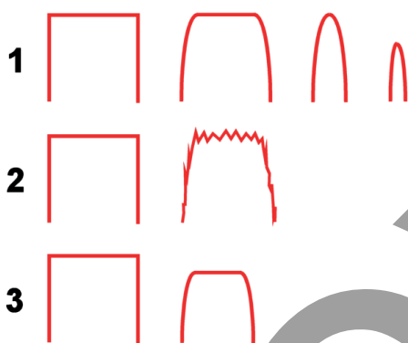
Figura 13: Modifiche dell'impulso elettrico
