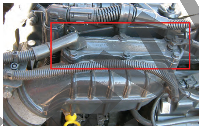
Figura 70: Collettore di aspirazione con resistenza di pre-riscaldamento
